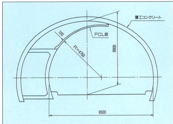
● 標準断面図
