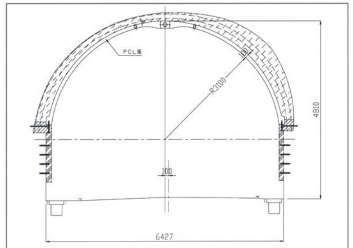
●標準断面図
