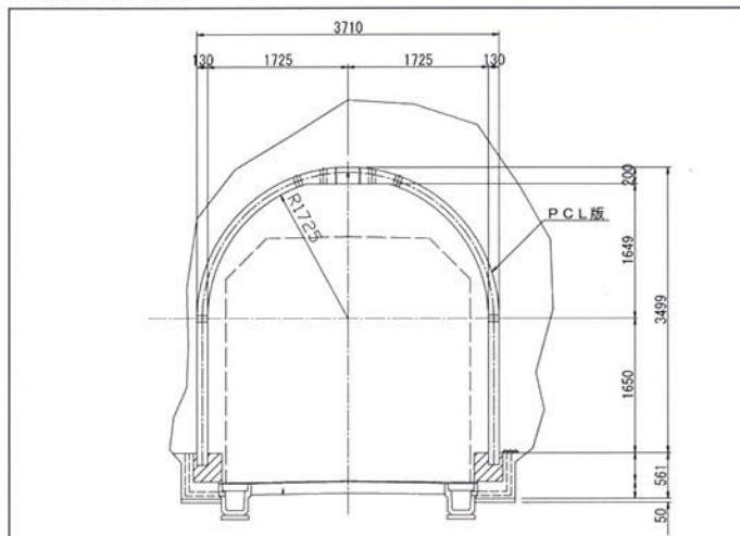
●標準断面図
