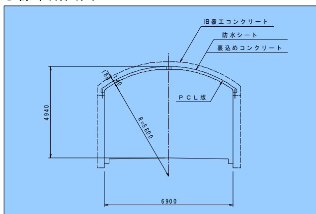
● 標準断面図
